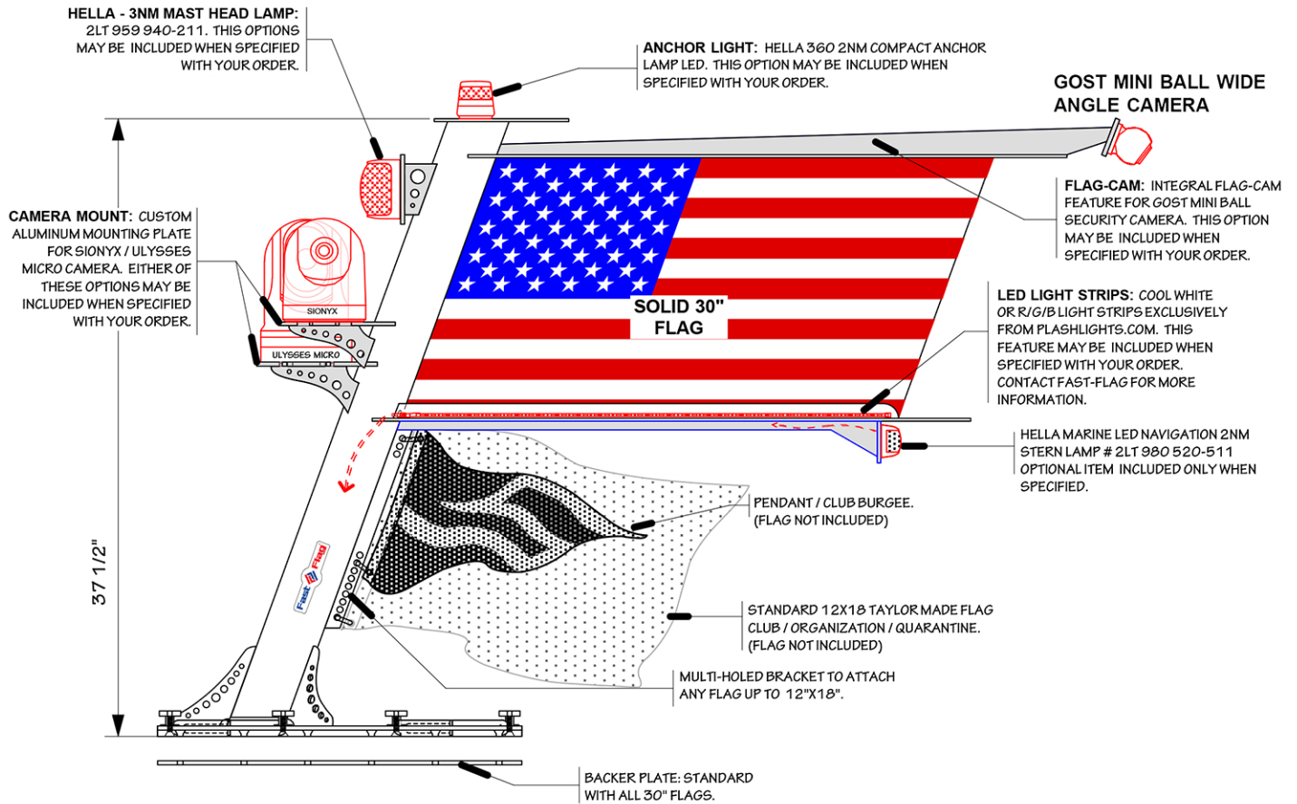
SSB-30FDB SOLID (PORT SIDE VIEW)
