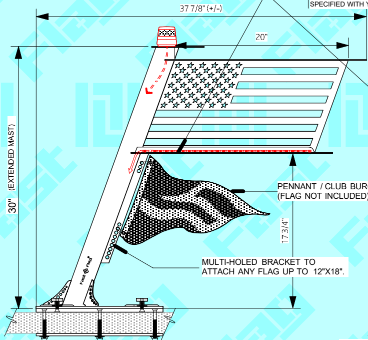
SSB-20FDB STENCIL
